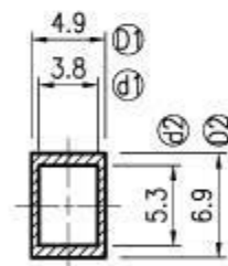
A-A Section
